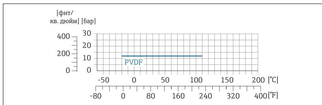
28 С материалом обжимного фитинга 1.4404/F316L/F316
