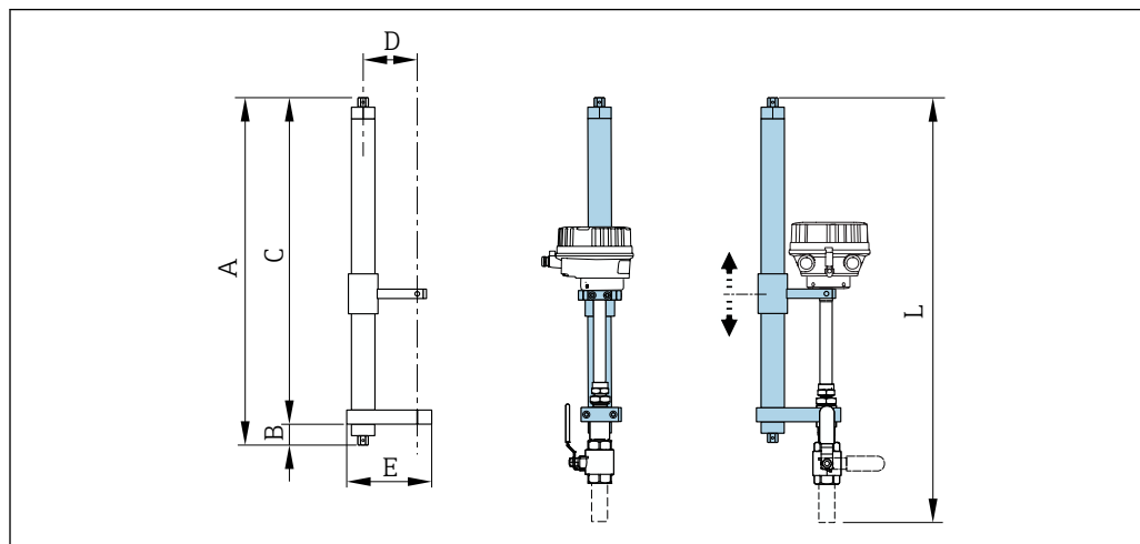
38 Экстрактор в сборе
