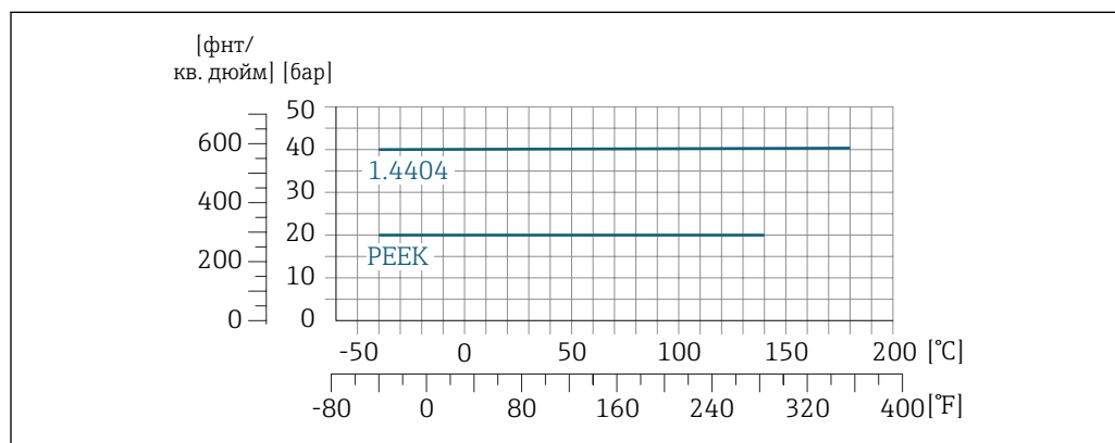
27 С материалом обжимного фитинга 1.4404/F316L/F316
