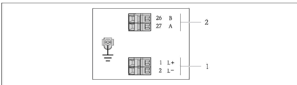
3 Назначение контактов PROFIBUS DP
