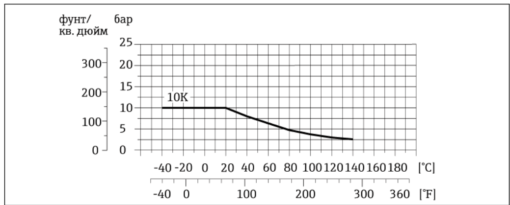
23 Присоединение к процессу, материал: PVDF
