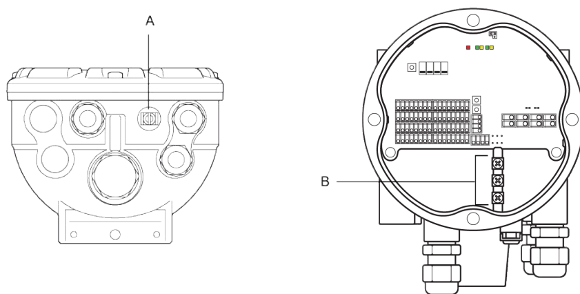
Рис. 4–2. Клеммы заземления
