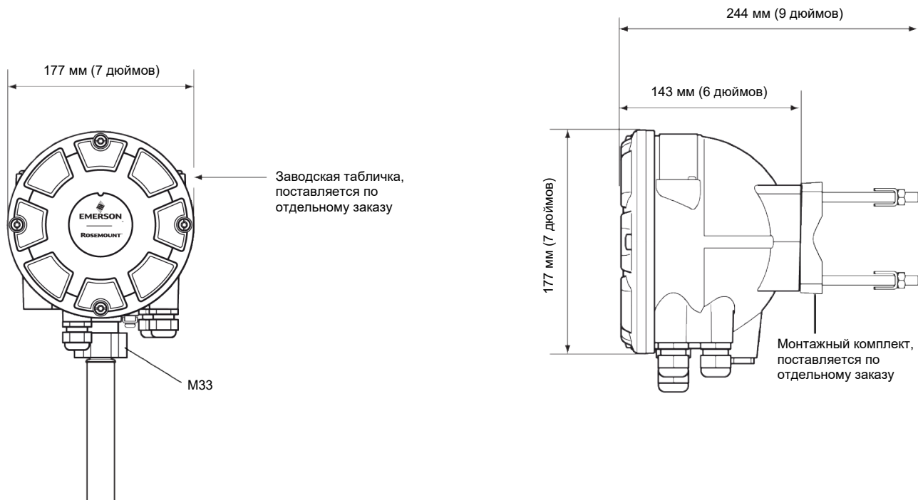
Рис. А-1. Размеры преобразователя температуры Rosemount 2240S
