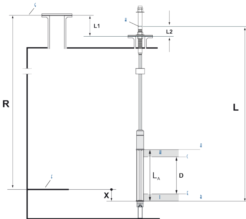
Рис. 5–7. Диапазон измерений и параметры отсчета
