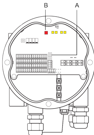
Рис. 5–3. Кнопка ZERO и сигнал состояния светодиодного индикатора
