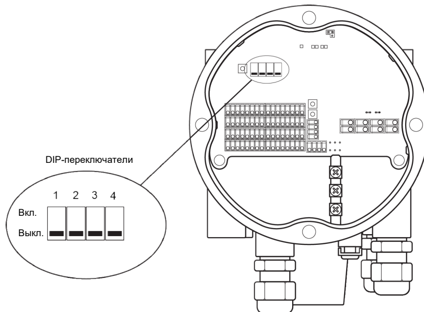
Рис. 5–10. DIP-переключатели
