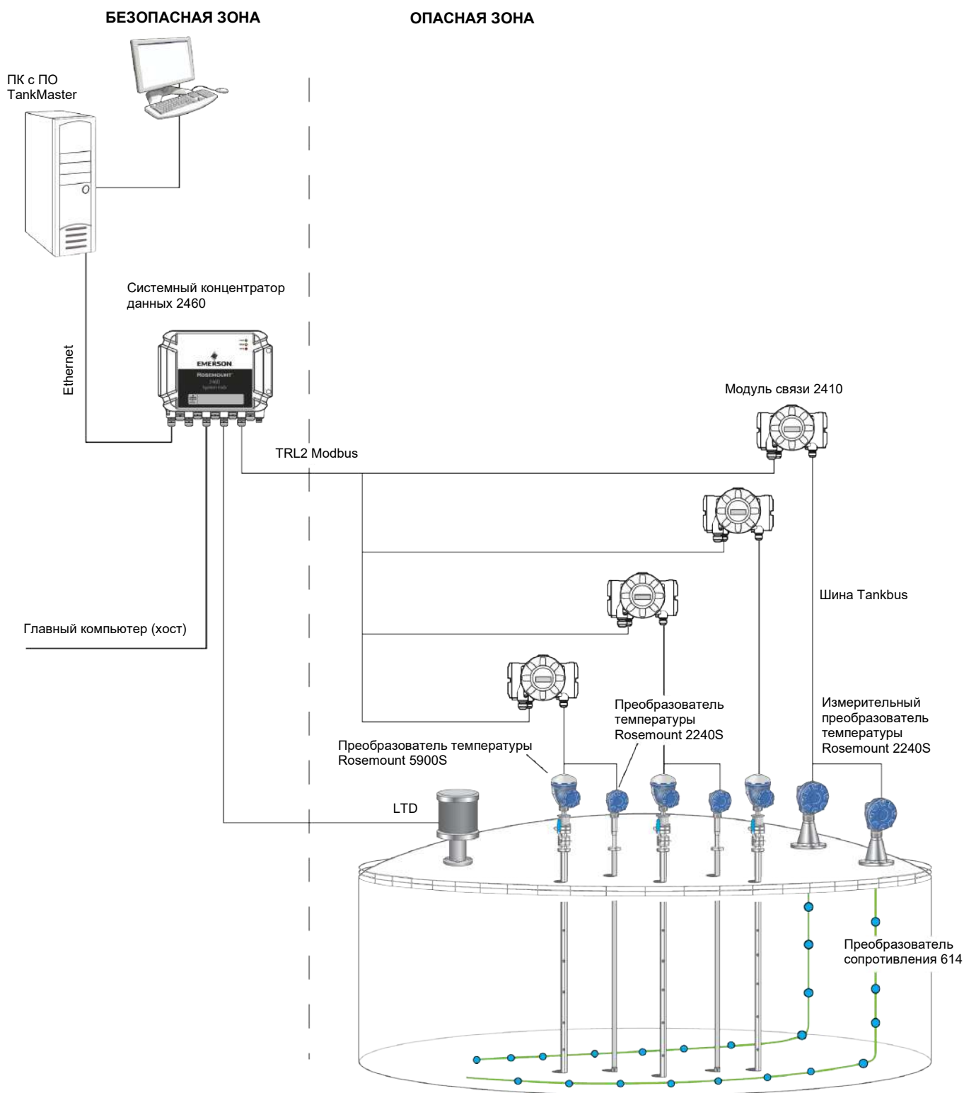
Рис. 2–6. Система измерительная для учета жидкостей в резервуарах Rosemount для резервуаров хранения сжиженных углеводородов (СПГ, СНГ)
