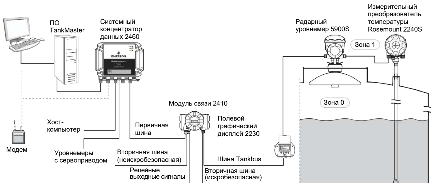
Рис. 2–1. Построение системы
