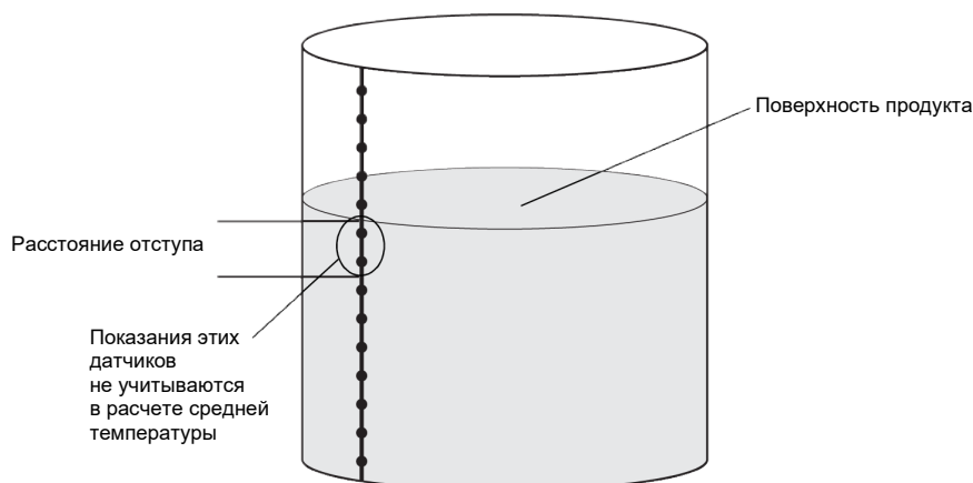
Рис. 5–2. Расстояние отступа
