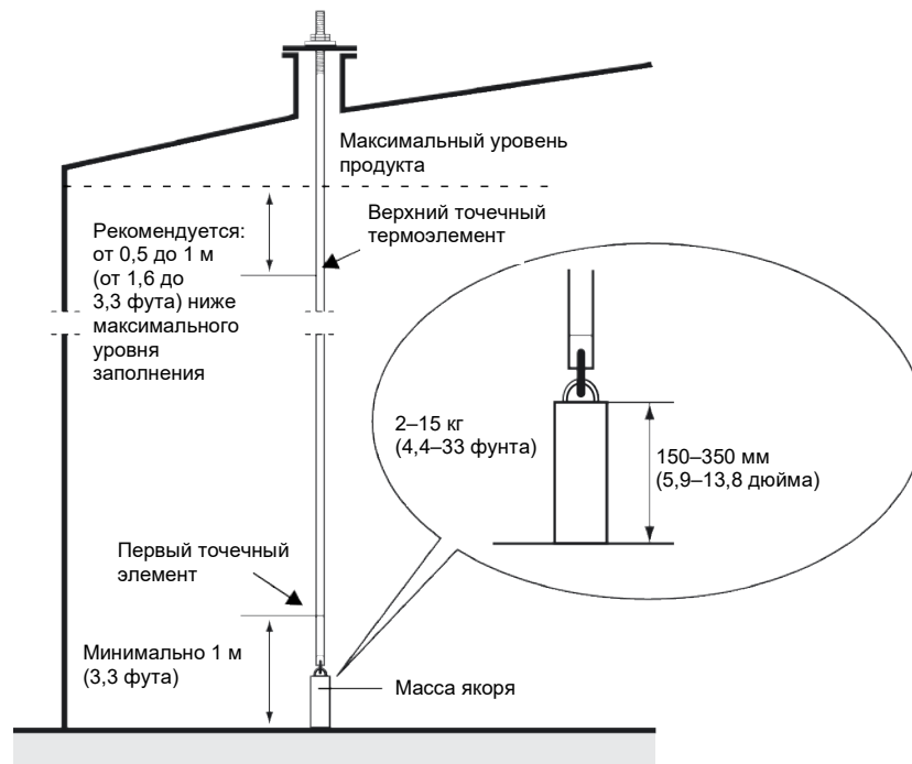
Рис. 3–1. Установка многоточечного датчика температуры в резервуарах со стационарной крышей
