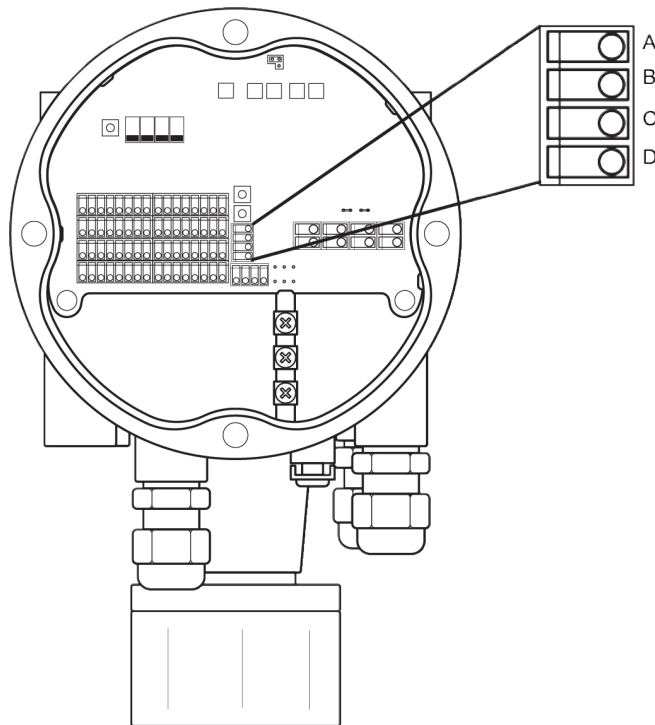
Рис. 6–5. Контрольная клемма для термоэлементов
