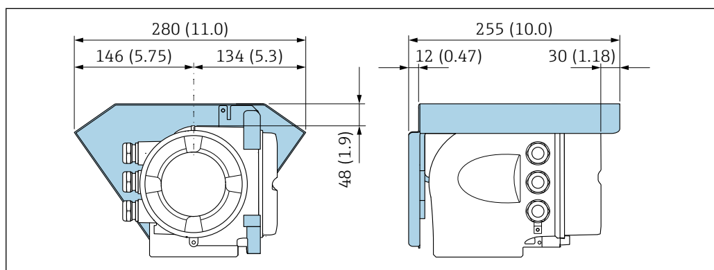
9 Защитный козырек для прибора Proline 500; единицы измерения – мм (дюймы)
