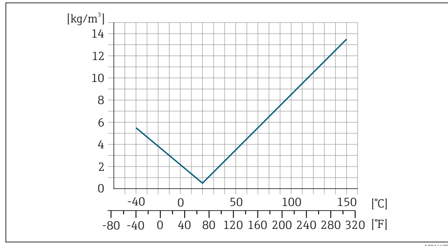
3 Калибровка по плотности на месте эксплуатации, в примере при +20 °C (+68 °F)
