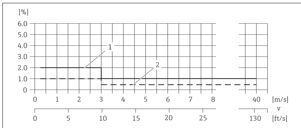
35 Пример максимальной погрешности измерения (объемный расход) в % от ИЗМ
