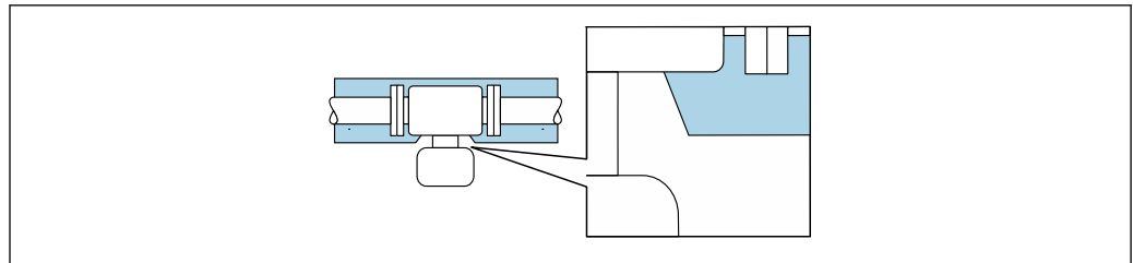
8 Теплоизоляция с открытой удлинительной шейкой
