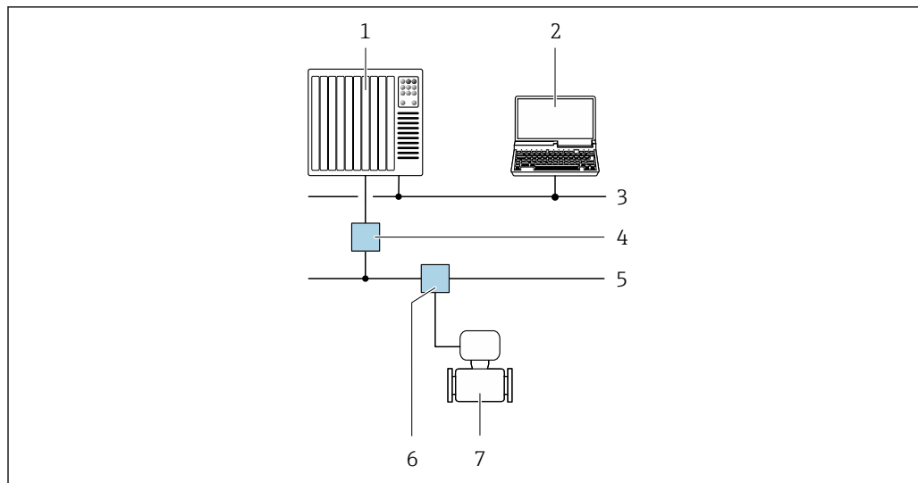
30 Варианты дистанционной работы через сеть PROFIBUS PA
