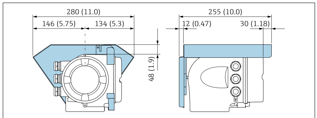
10 Защитный козырек для прибора Proline 500; единицы измерения – мм (дюймы)
