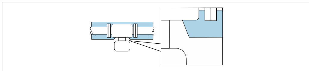
19 Теплоизоляция с открытой удлинительной шейкой
