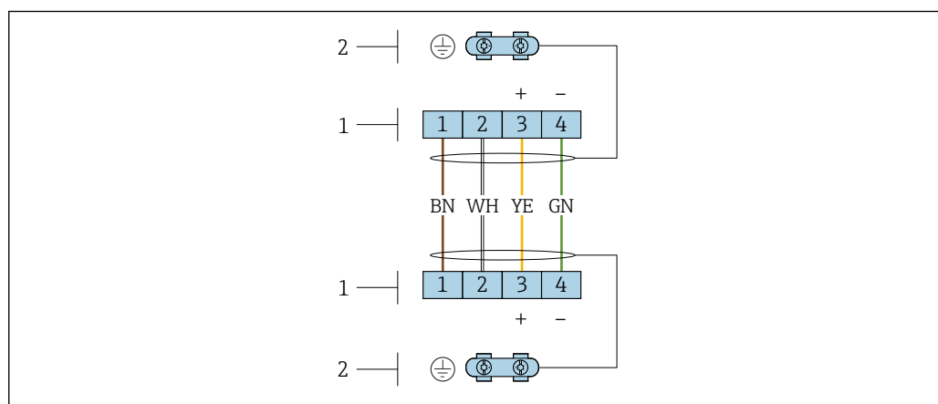
11 Клеммы для клеммного отсека, расположенного в настенном держателе электронного преобразователя, и для клеммного отсека датчика
