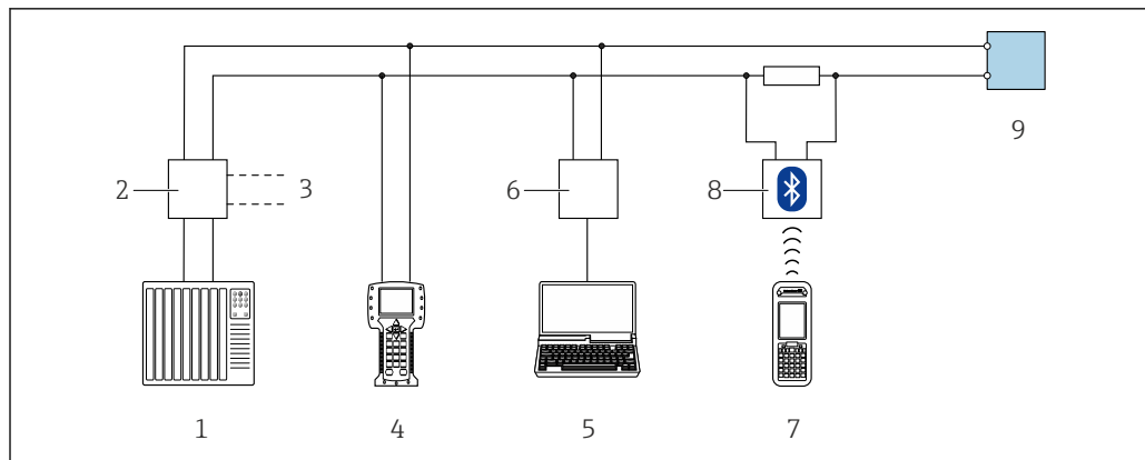
19 Варианты дистанционного управления по протоколу HART (пассивный режим)
