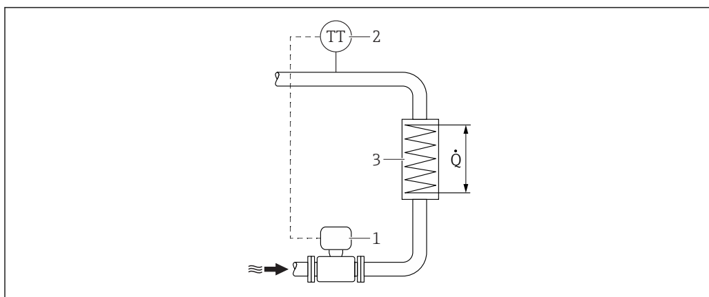
7 Схема измерения изменения количества теплоты для насыщенного пара и воды
