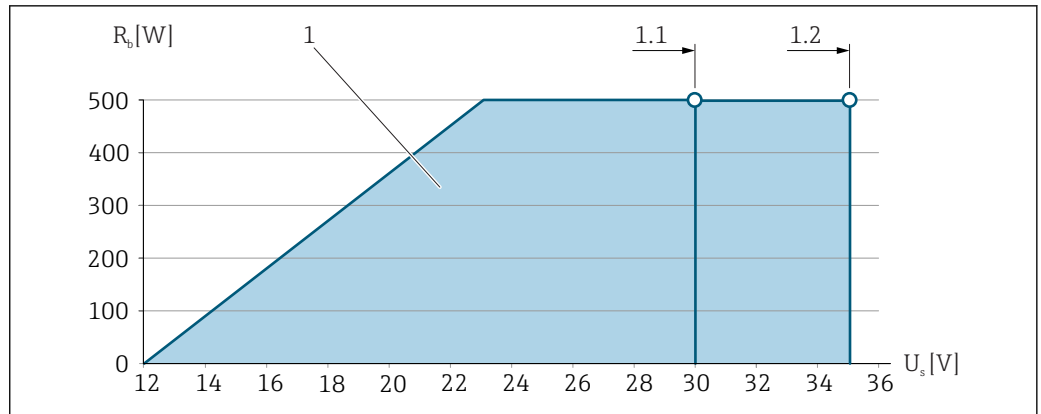
12 Нагрузка для компактного исполнения без локального управления
