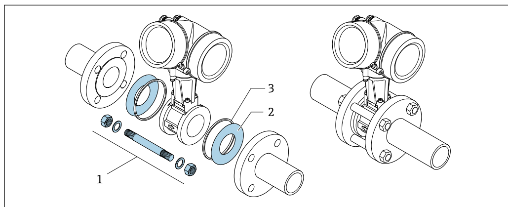
8 Монтажный комплект для бесфланцевого исполнения
