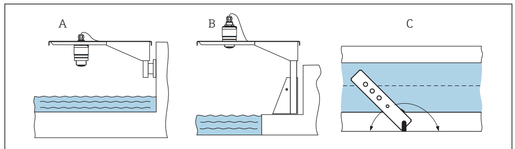
12 Монтаж на кронштейне, с возможностью поворота
