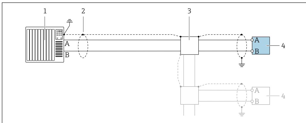
8 Пример подключения для Modbus RS485, невзрывоопасная зона и зона 2; класс I, раздел 2
