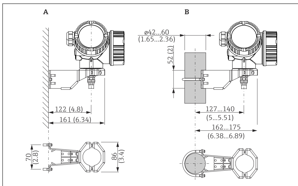
7 Монтаж корпуса электронной части с использованием кронштейна; размеры: мм (дюйм)
