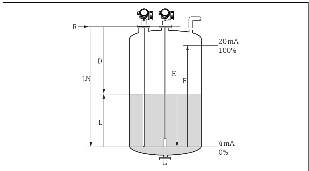
26 Параметры конфигурации для измерения уровня в жидкостях
