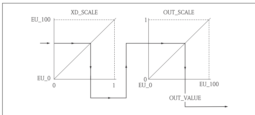
25 Масштабирование измеренного значения в блоке AI
