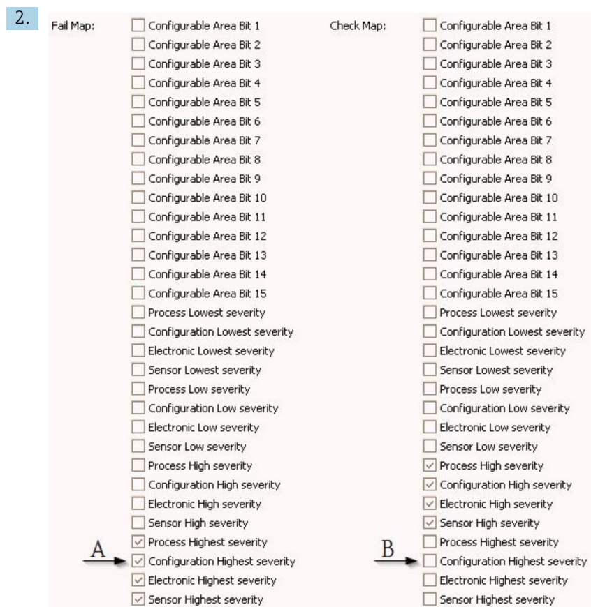
27 Стандартное состояние столбцов «Карта неисправностей» и «Карта проверок»
