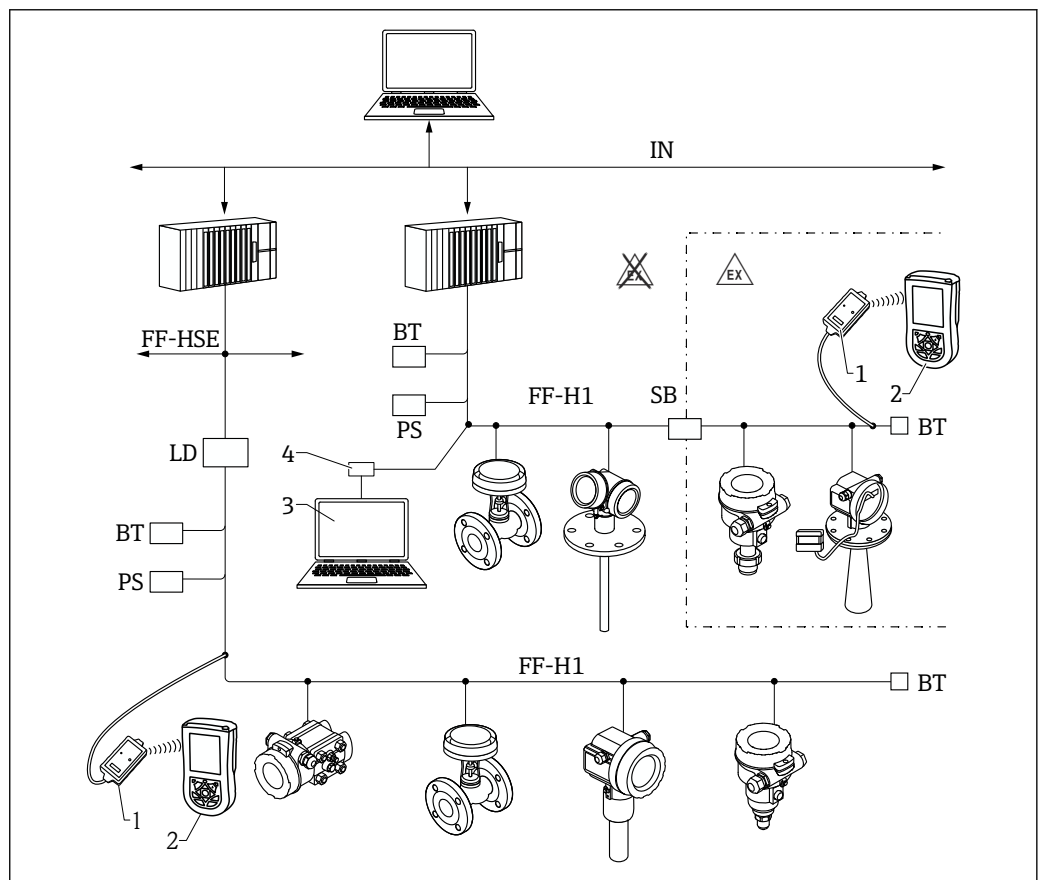
17 Системная архитектура FOUNDATION Fieldbus и сопутствующие компоненты
