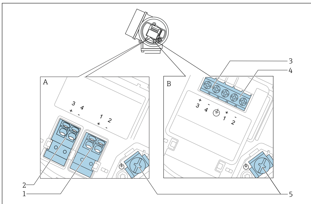
10 Назначение клемм; PROFIBUS PA/FOUNDATION Fieldbus
