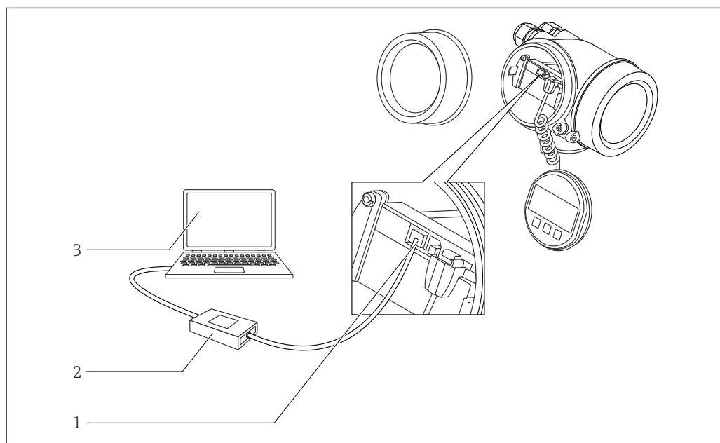
18 DeviceCare/FieldCare через сервисный интерфейс (CDI)
