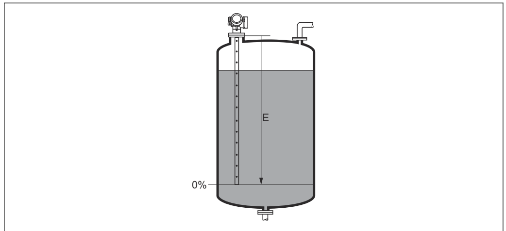
34 Калибровка пустой емкости (E) для измерения уровня жидких сред
