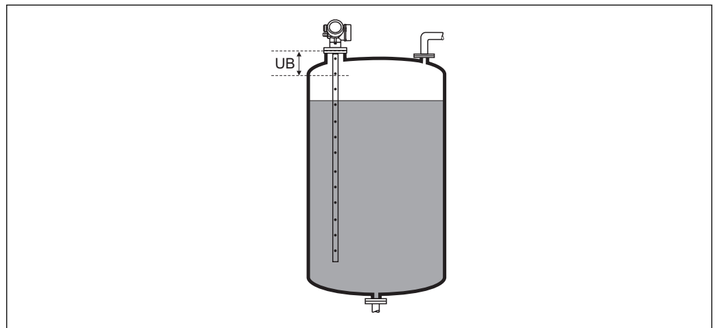
46 Блокирующая дистанция (UB) для измерения в жидких средах
