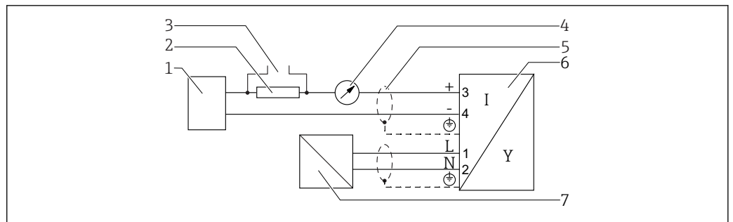
16 Блок-схема 4-проводного подключения: 4–20 мА HART (90 до 253 V AC )
