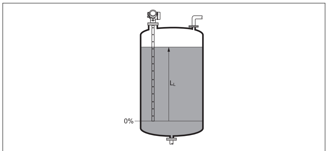
41 Уровень при измерении в жидких средах
