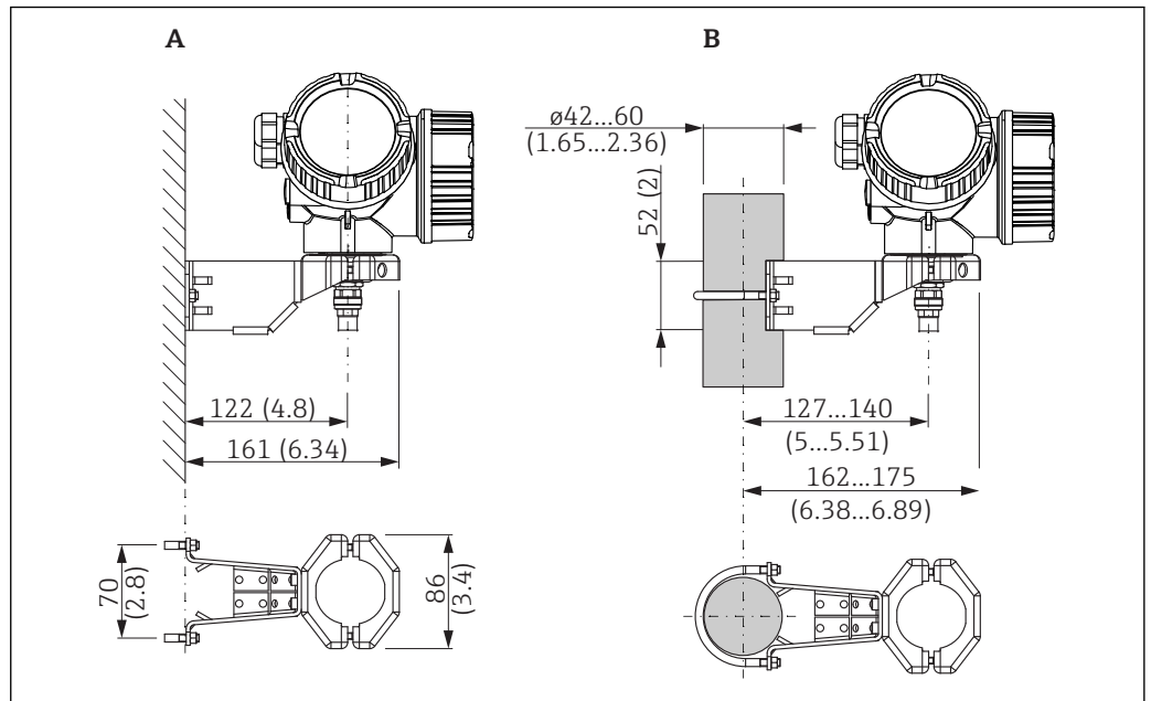
6 Монтаж корпуса электроники на монтажном кронштейне. Единица измерения мм (дюйм)
