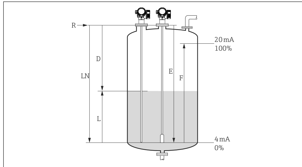
33 Параметры конфигурации для измерения уровня жидких сред
