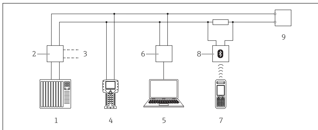
▣ 26 Варианты дистанционного управления по протоколу HART
