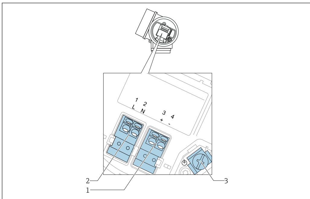
15 Назначение клемм, 4-проводное подключение; 4–20 мА HART (90 до 253 V AC )
