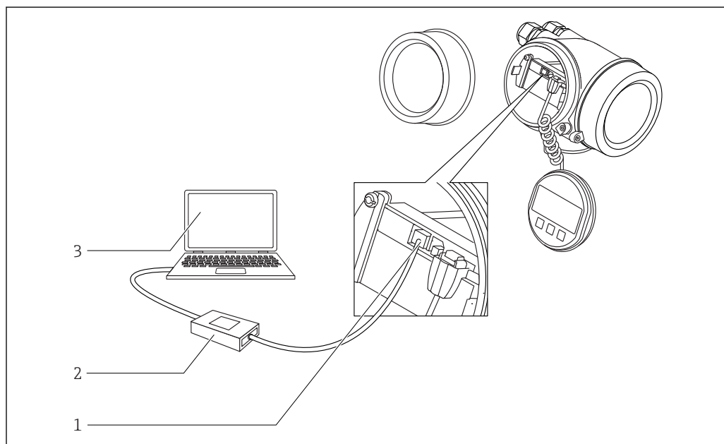
▣ 27 DeviceCare/FieldCare через сервисный интерфейс (CDI)
