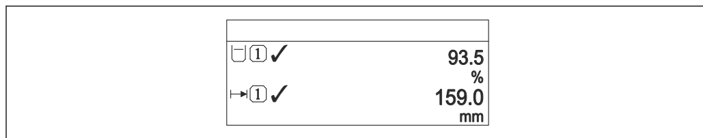
49 «Форматировать дисплей» = «2 значения»
