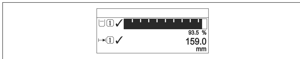
48 «Форматировать дисплей» = «1 гистограмма + 1 значение»
