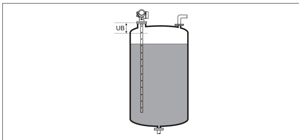
43 Блокирующая дистанция (UB) для измерения в жидких средах
